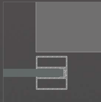
Schiebetür ohne Zarge
