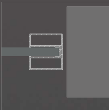
Pendeltür ohne Zarge
